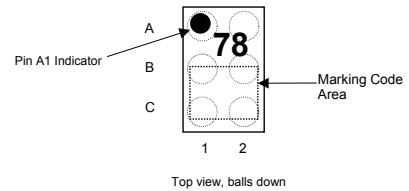
IP4078CX6/LF outline dimensions
